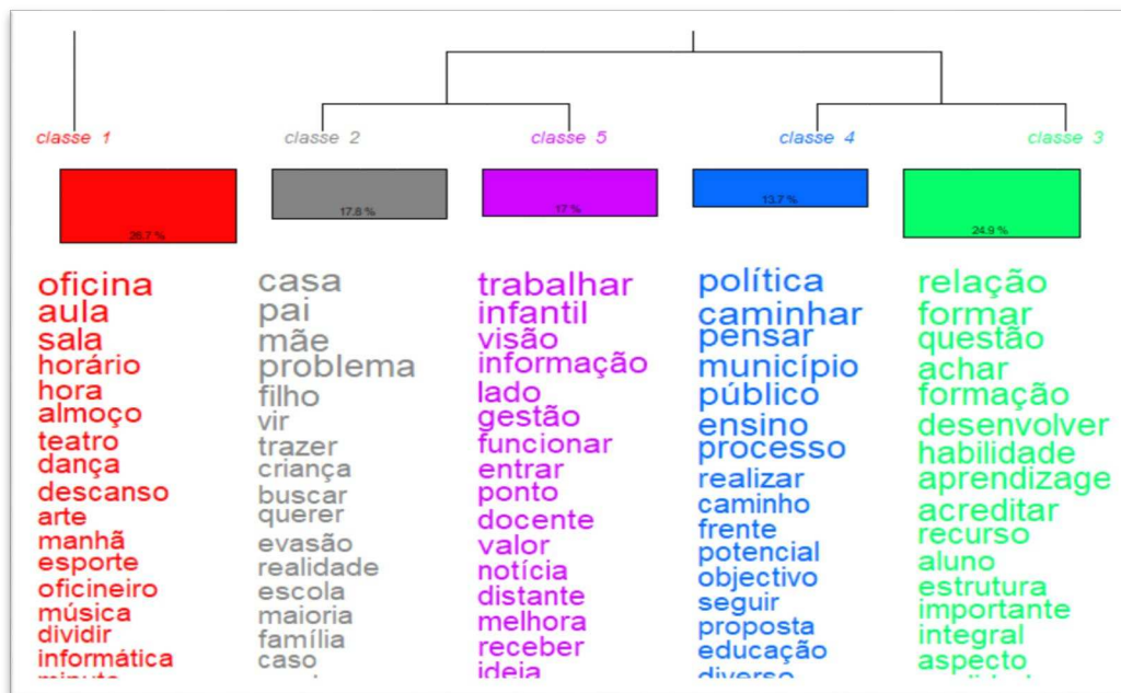
Figura 1: Dendrograma - entrevistas
